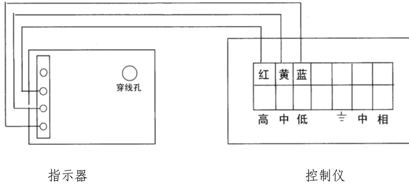
图3 接线图
