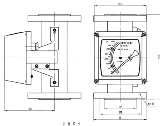
图 4 安装尺寸
