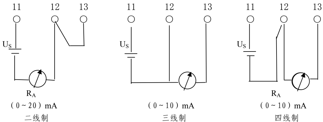
图 2 接线图
